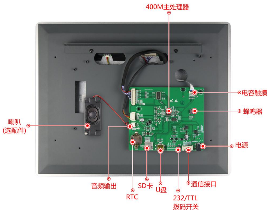
图 1-2 硬件配置图
