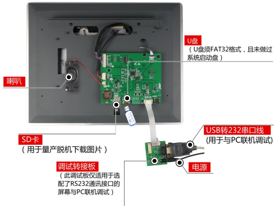
图 1-3 RS232 调试工具图
